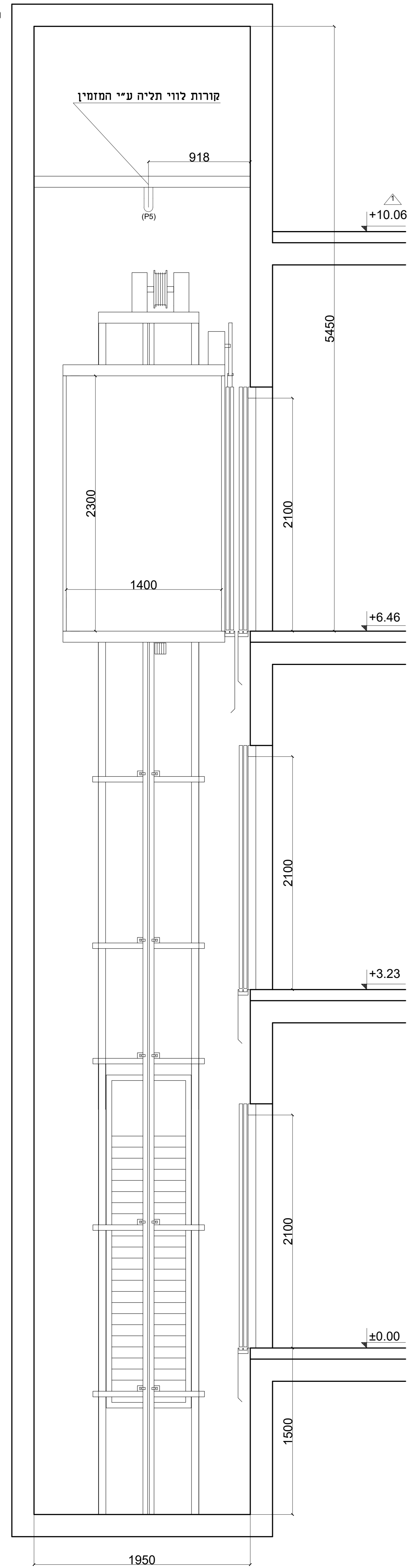
חתך - כללי א - א
