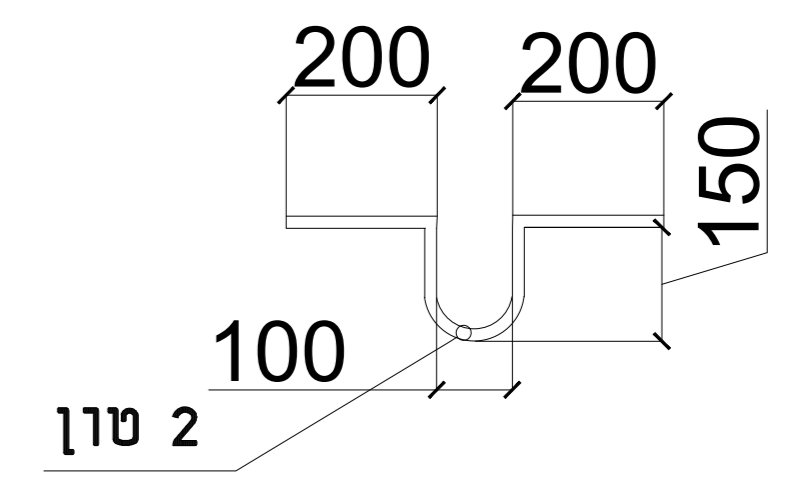
פרט וו בתקרה
