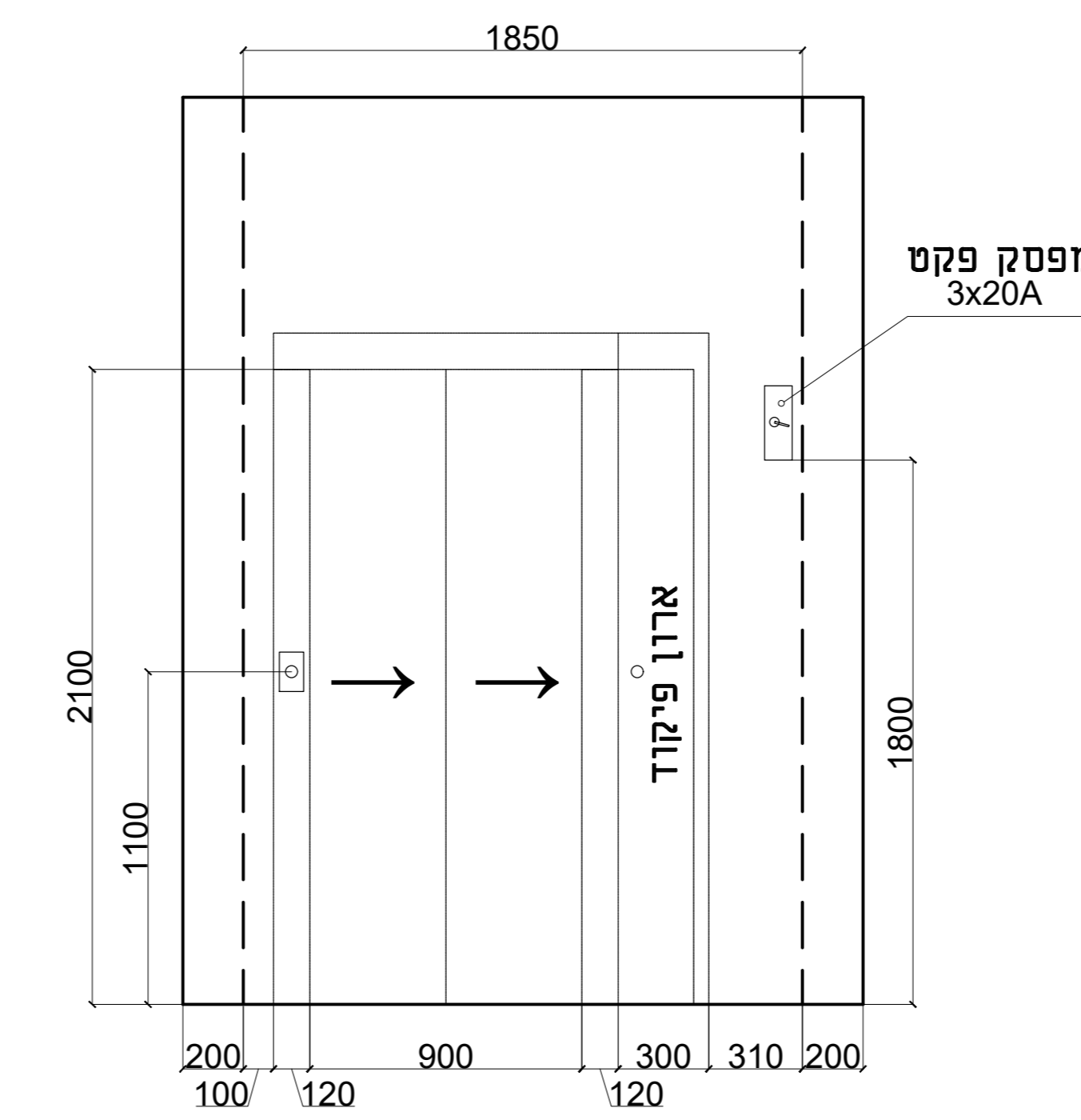
חזית - כללי תחנה עליונה בלבד
